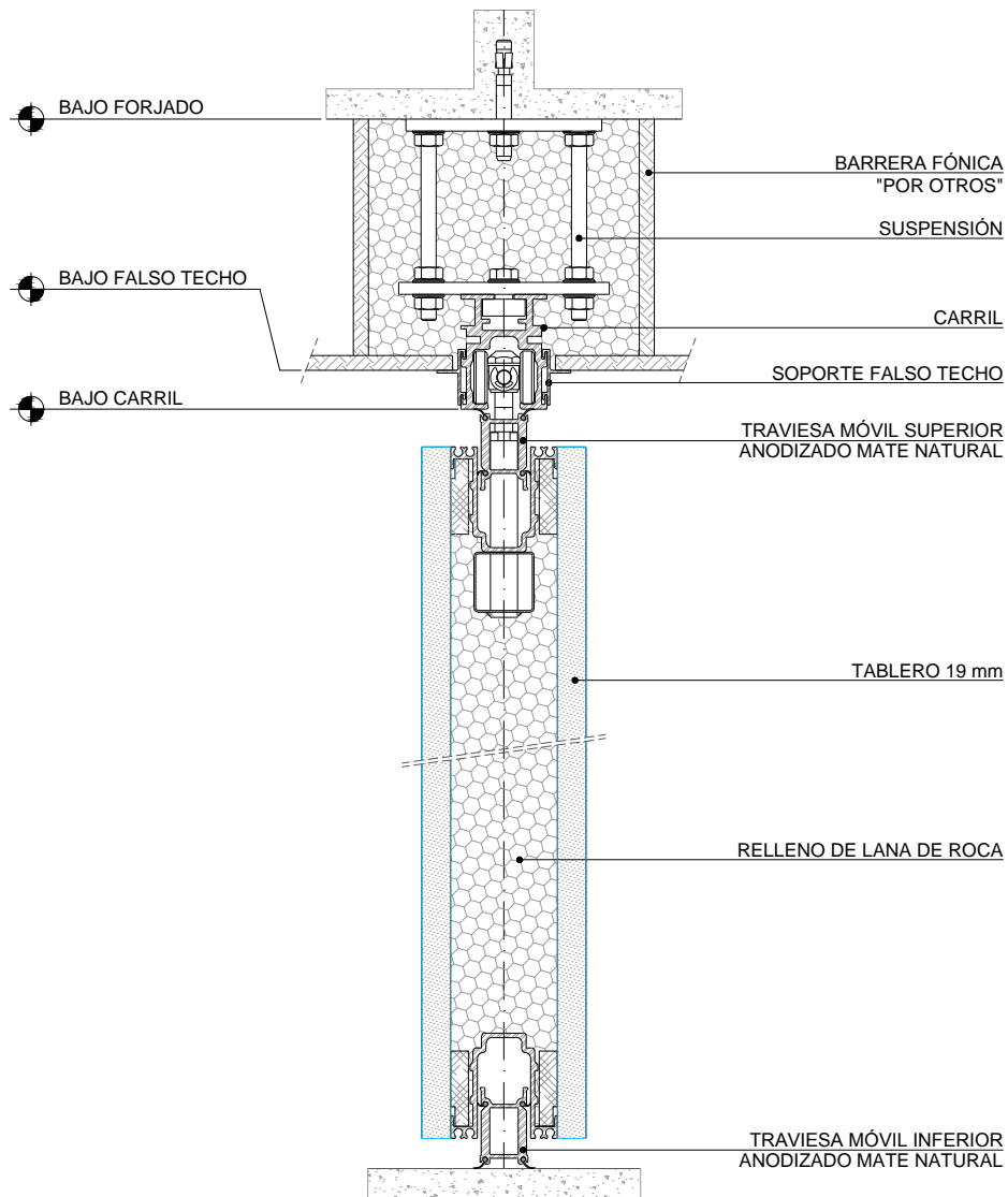
SECCIÓN VERTICAL
